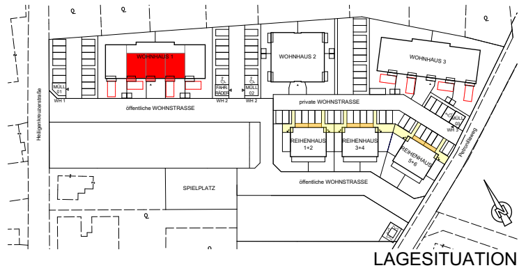
LAGESITUATION
