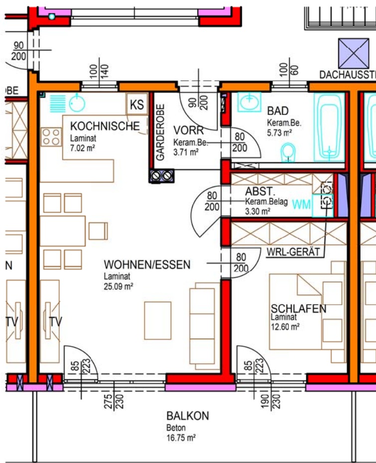
Grundriss Top 6 / Top 7 spiegelbildlich
