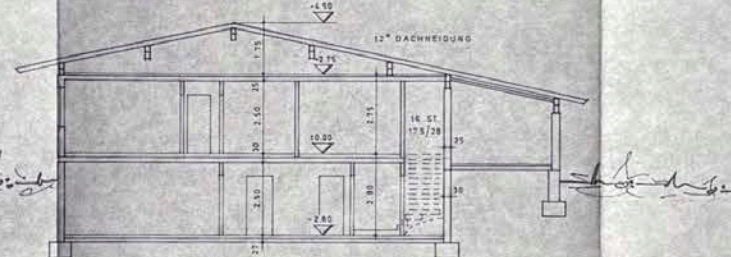
schnitt
