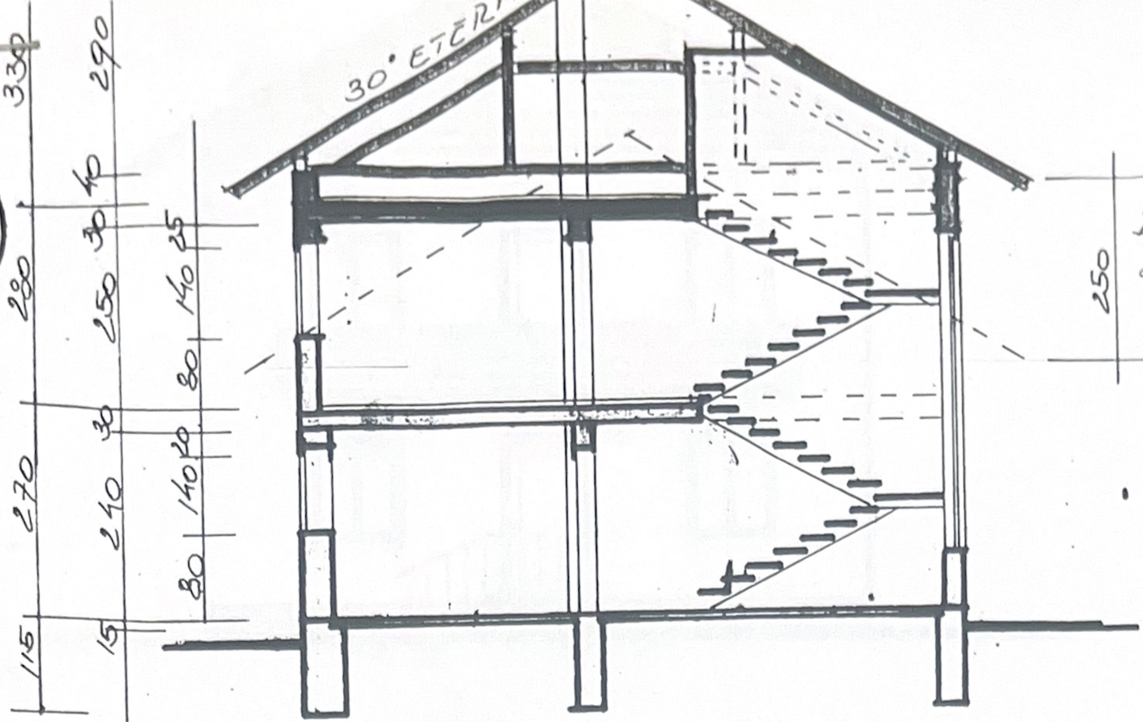
SCHNITT A-A
