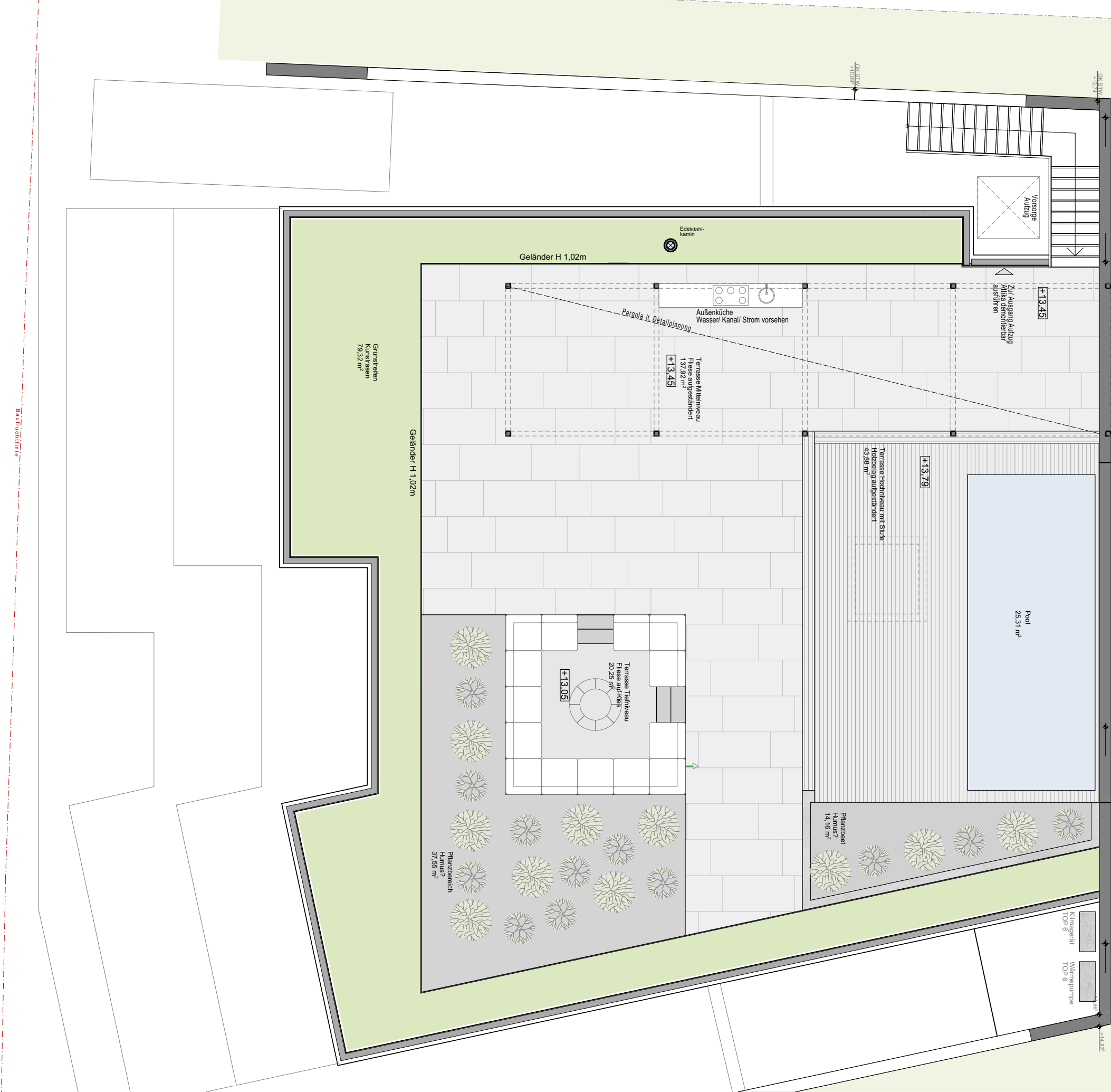
KUNDENPLAN TOP 6 DACHTERRASSE
