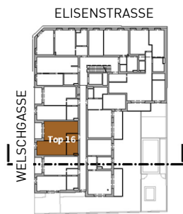
GRUNDRISS (2.OG)
