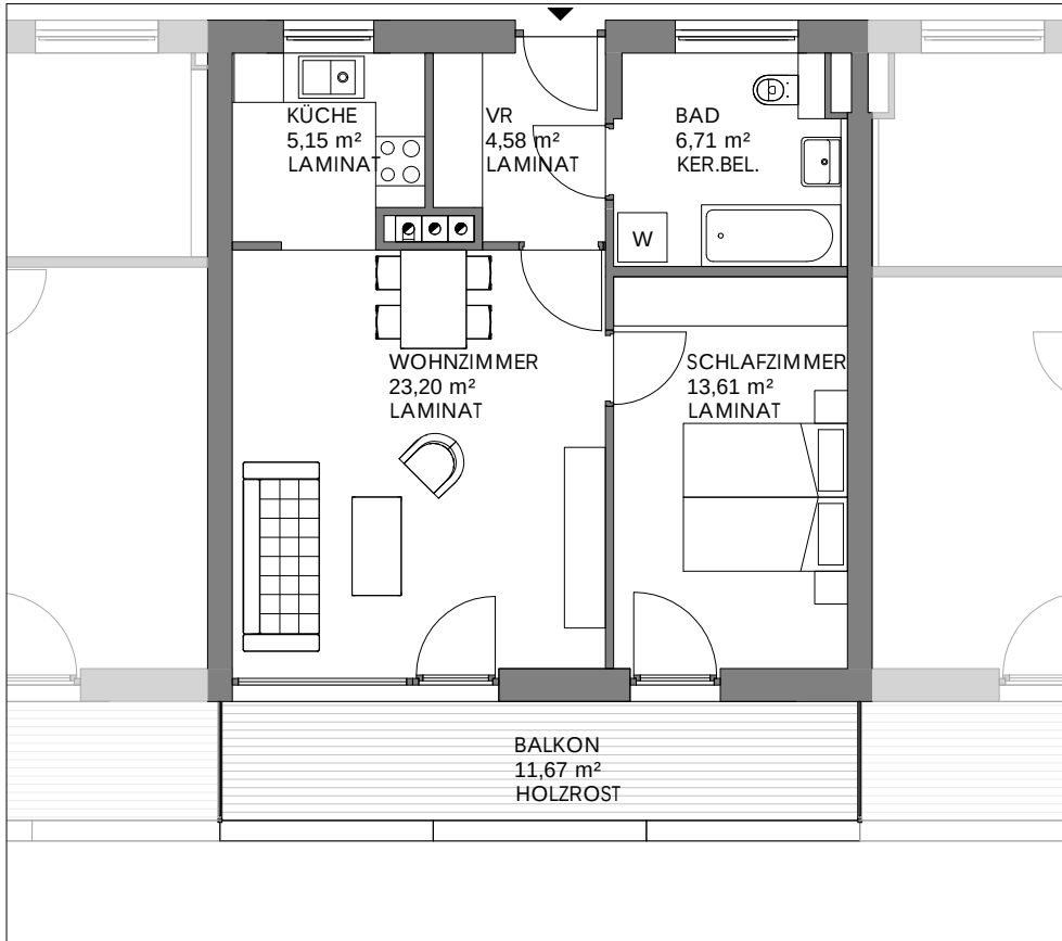
GRUNDRISS WOHNUNG M 1:100
