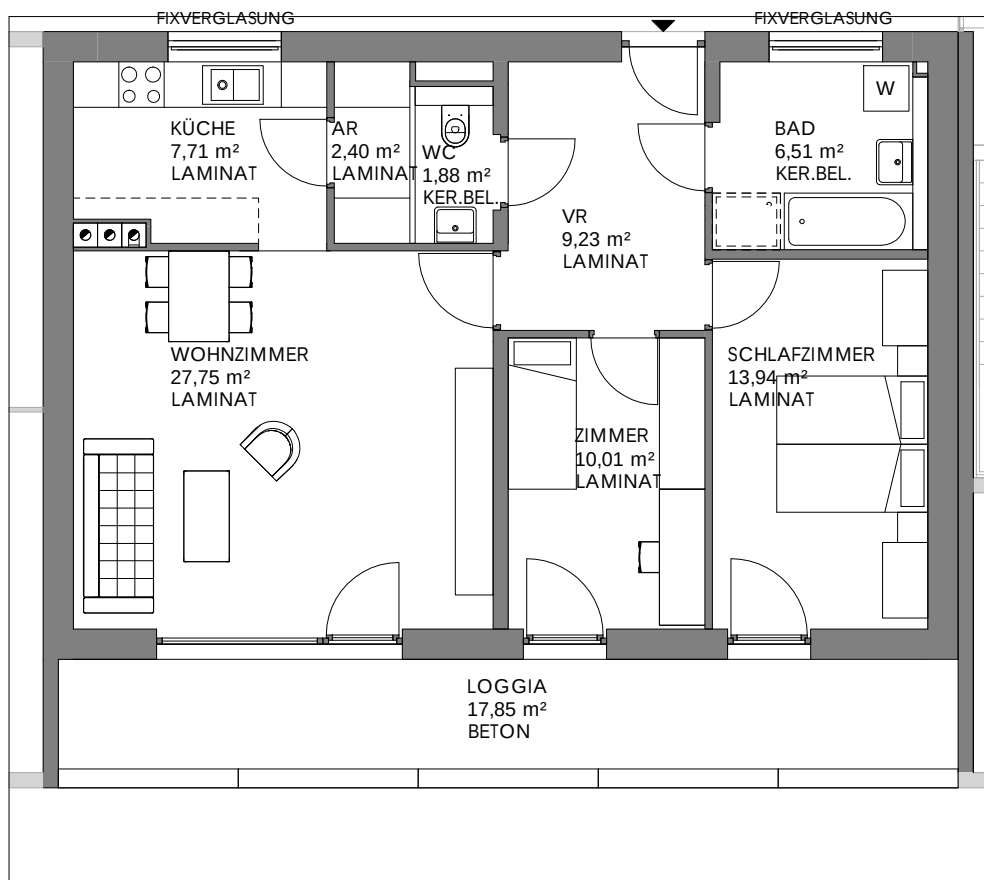
GRUNDRISS WOHNUNG M 1:1000
