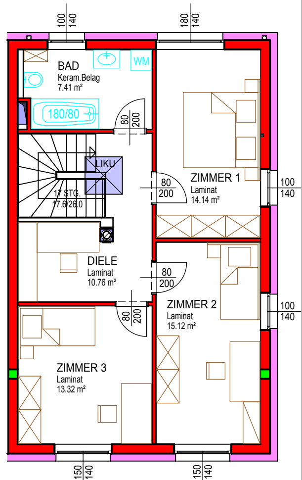
Obergeschoss
