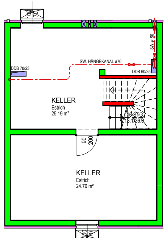
Kellergeschoss
