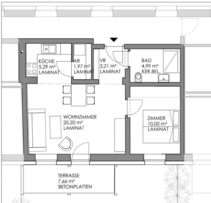
GRUNDRISS ERDGESCHOSS M 1:100
