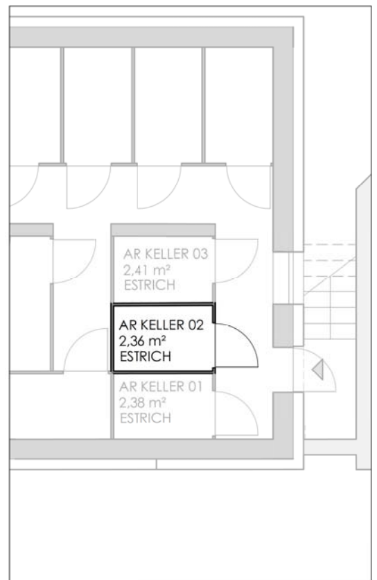
GRUNDRISS KELLER M 1:100
